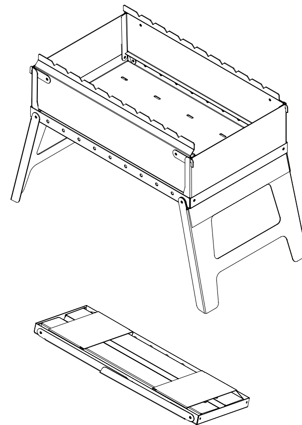
Рис. 2 - Схема мангала в собранном виде и в рабочем состоянии.
