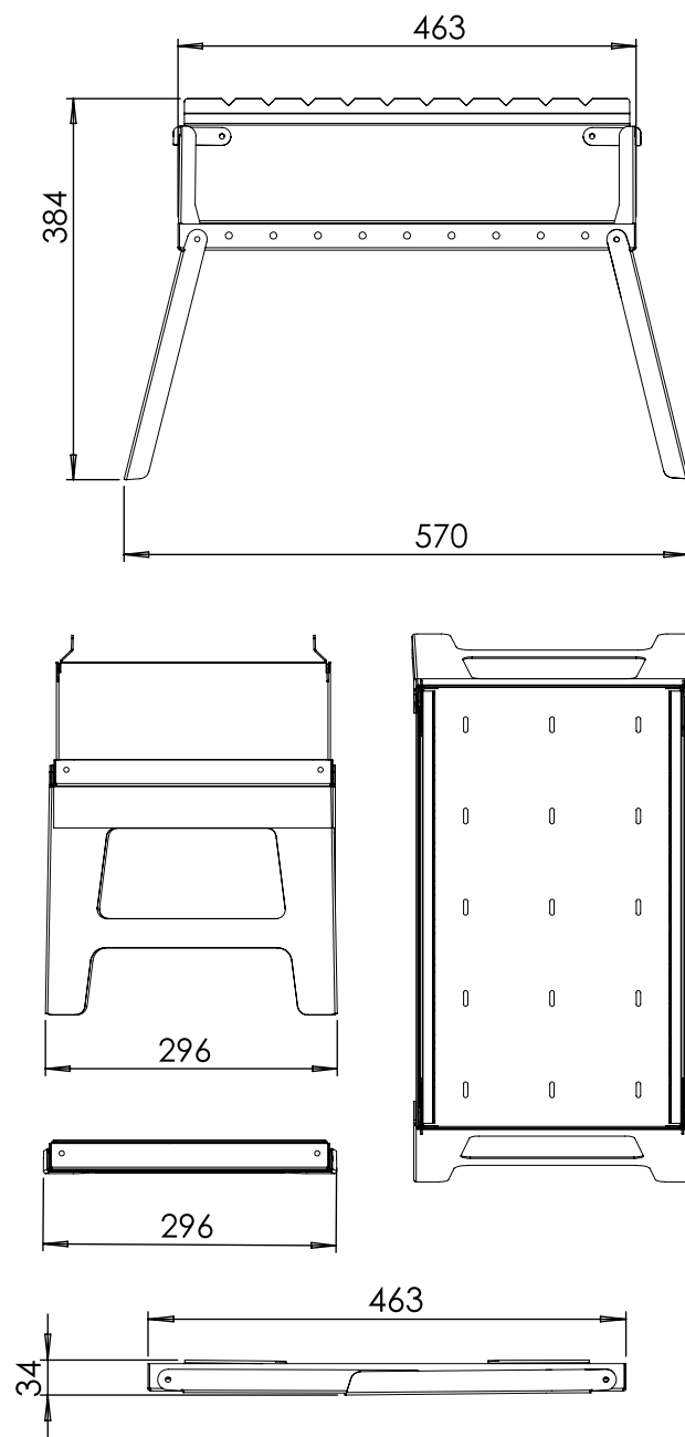
Рис. 1 - Габаритные размеры мангала.
