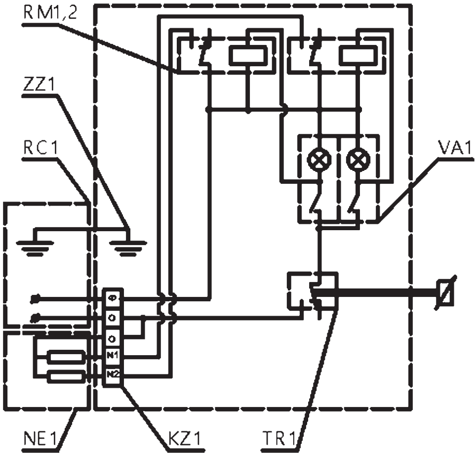
Рисунок 2 Схема ПУЭ-6
